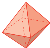
poliedro II
