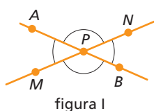
figura I
