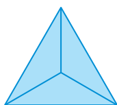
triângulo
