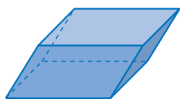
paralelepípedo oblíquo
