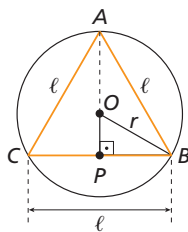
figura II
