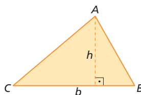
Figura I
