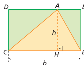
Figura II
