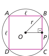
figura I
