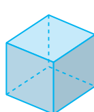
hexaedro regular (ou cubo)
