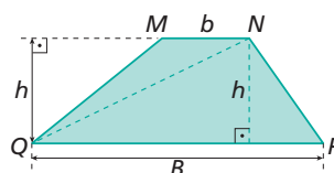
Figura II
