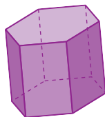
poliedro I
