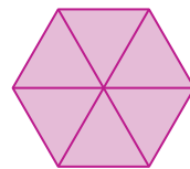
hexágono
