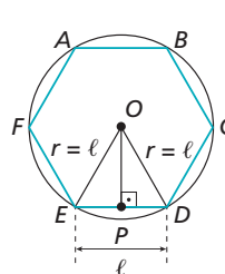
figura III
