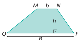
Figura I
