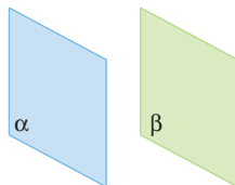
planos paralelos distintos (não coincidentes)
