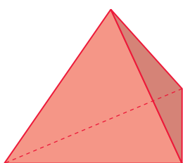
pirâmide triangular (tetraedro)
