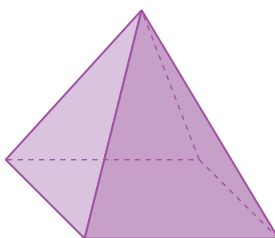
pirâmide quadrangular
