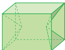
poliedro I
