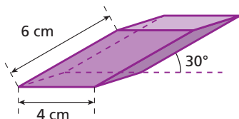
prisma oblíquo de base quadrada
