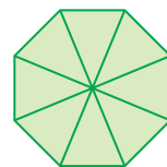
octógono
