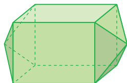
poliedro II
