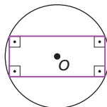
retângulo inscrito
