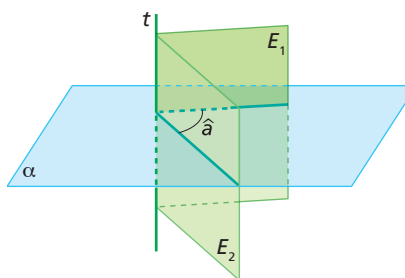
m(\hat{a}) é a medida do diedro E_1 \cup E_2
