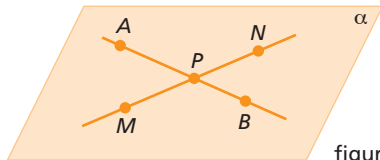
figura II
