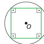
quadrado inscrito
