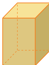
paralelepípedo reto-retângulo
